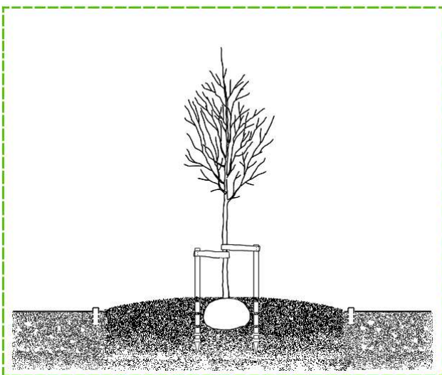
Figur 12. Upphöjd växtbädd när växtbäddens botten är mindre stabil. Ca 15 % sättning av en ditforslad eller djupluckrad jord är ett vanligt riktvärde.
